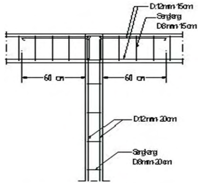
DETAIL HUBUNGAN BETON TANGKAI DENGAN RING BALOK
