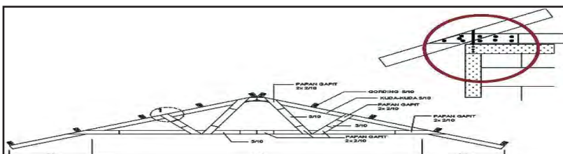
KUDA - KUDA KAYU 5/10 SEKALA 1 : 50
