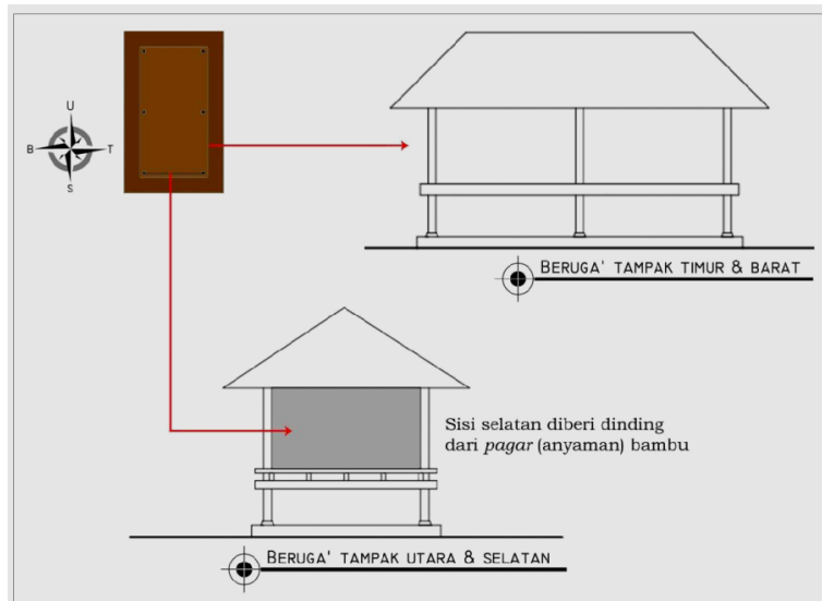
GAMBAR 5 ARSITEKTUR BERUGAQ SEKENEM
