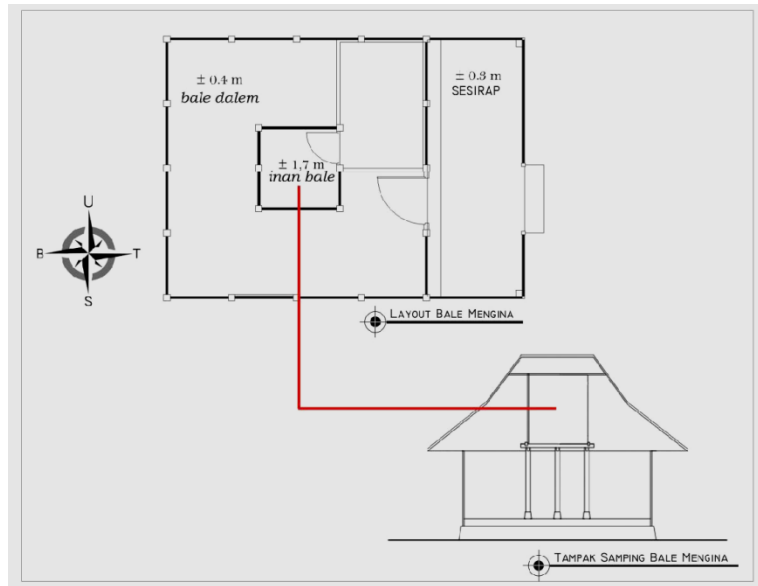
GAMBAR 4 ARSITEKTUR BANGUNAN BALE MENGINA
